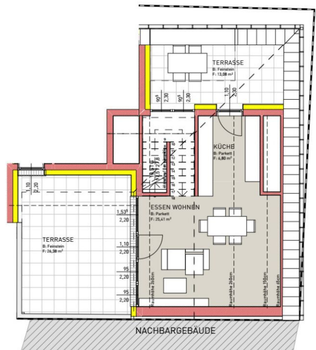
2.Obergeschoss
